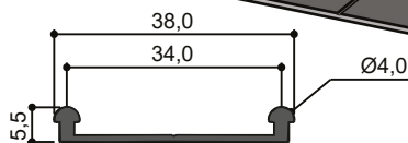
Trilho concavo 34
