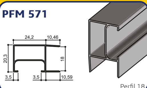
Perfil 18
