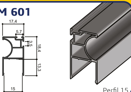
Perfil 15
