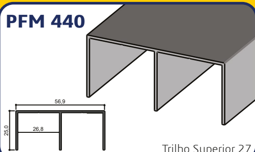
Trilho Superior 27
