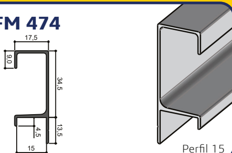
Perfil 15
