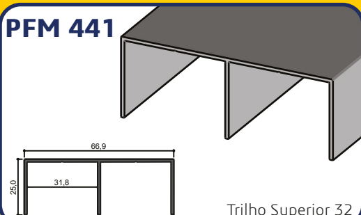
Trilho Superior 32
