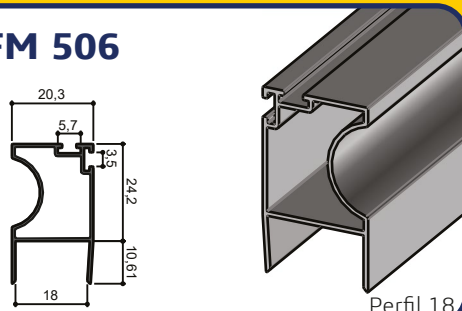
Perfil 18
