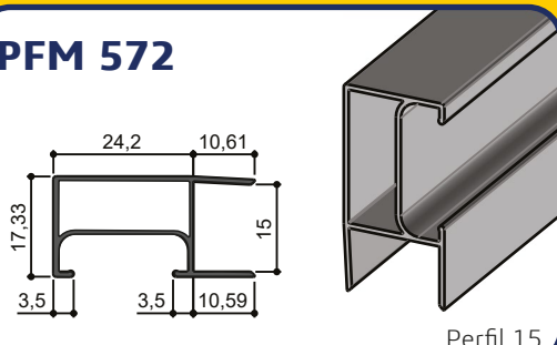
Perfil 15
