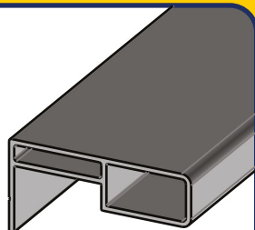
Perfil 18
